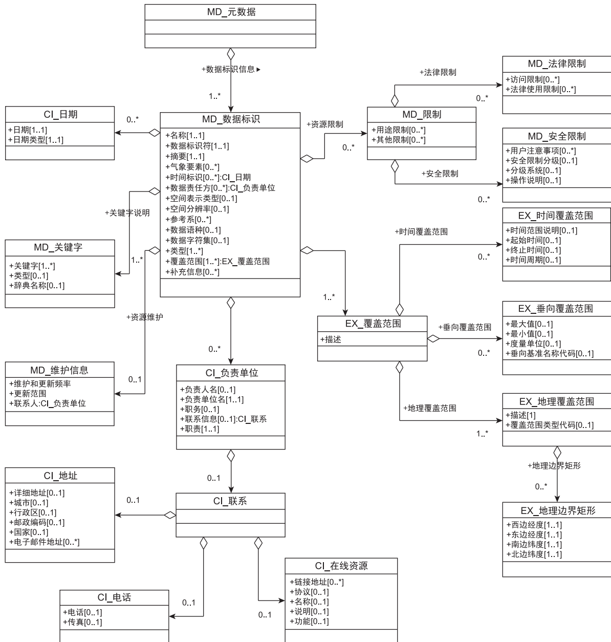
图 2 数据标识信息
