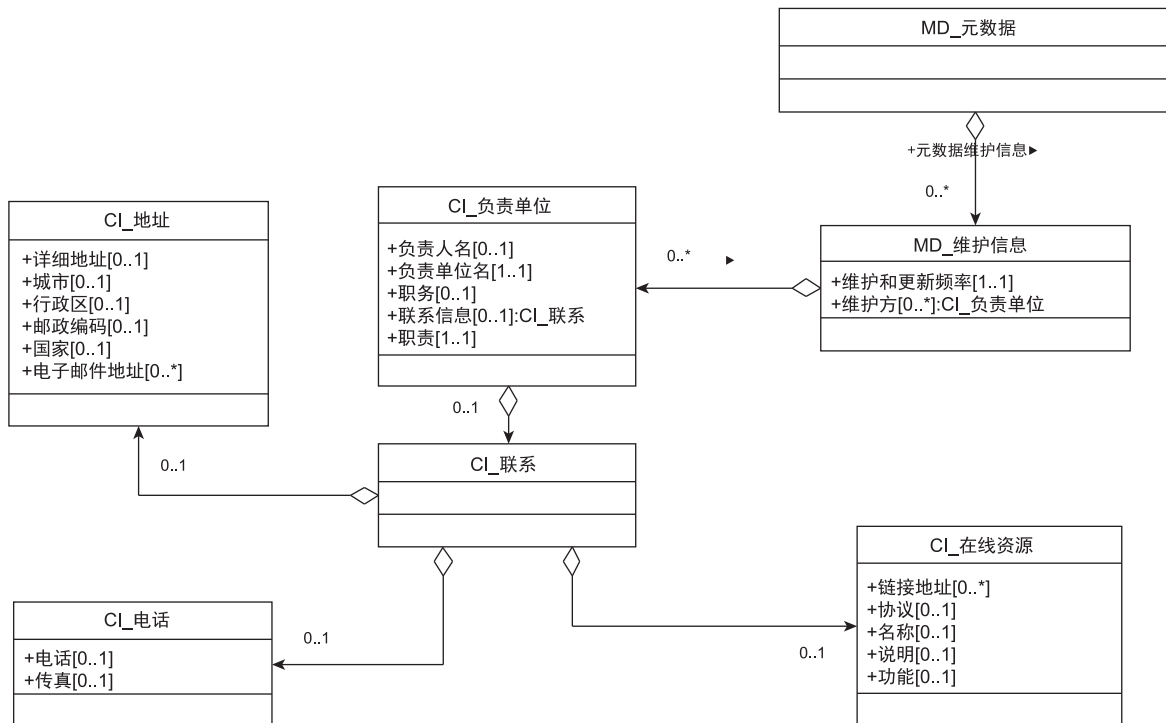
图 6 元数据维护信息
