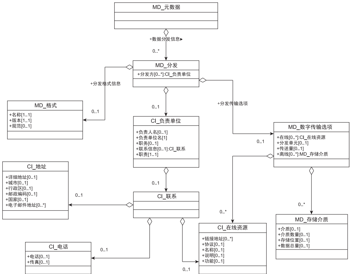
图 3 数据分发信息
