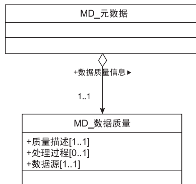
图 4 数据质量信息
