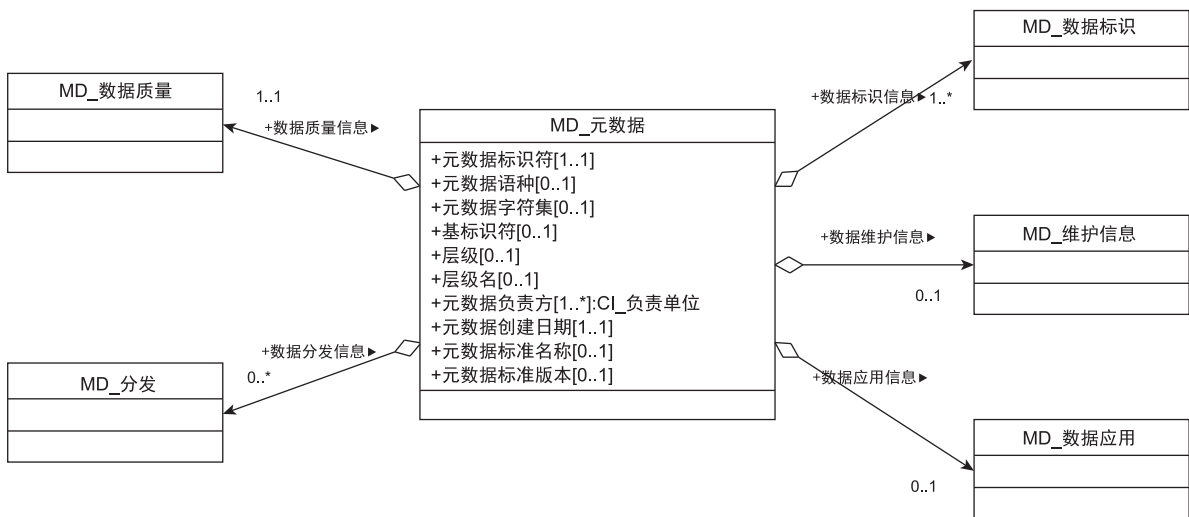
图 1 元数据实体集信息
