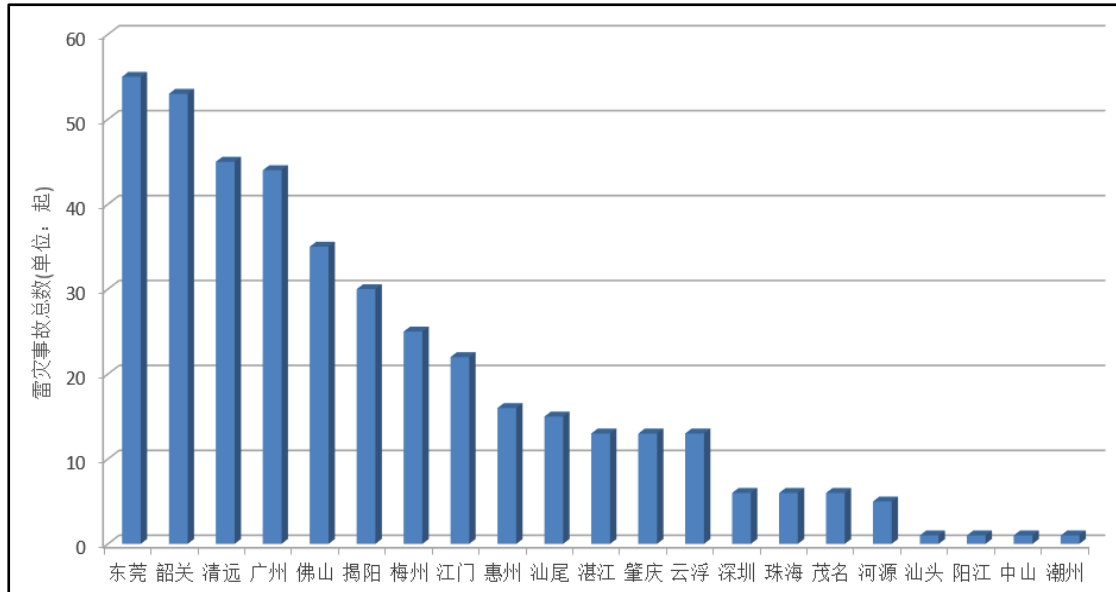
2016年各地市雷灾事故总数分布图
