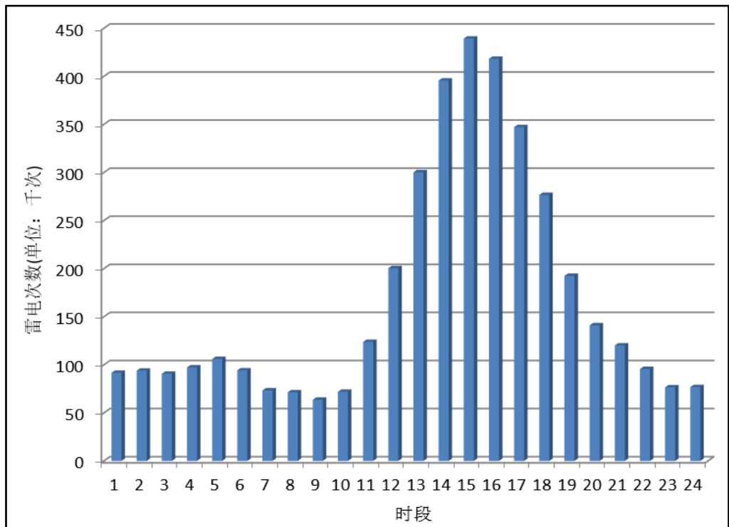
2016 年全省雷电活动时分布图
