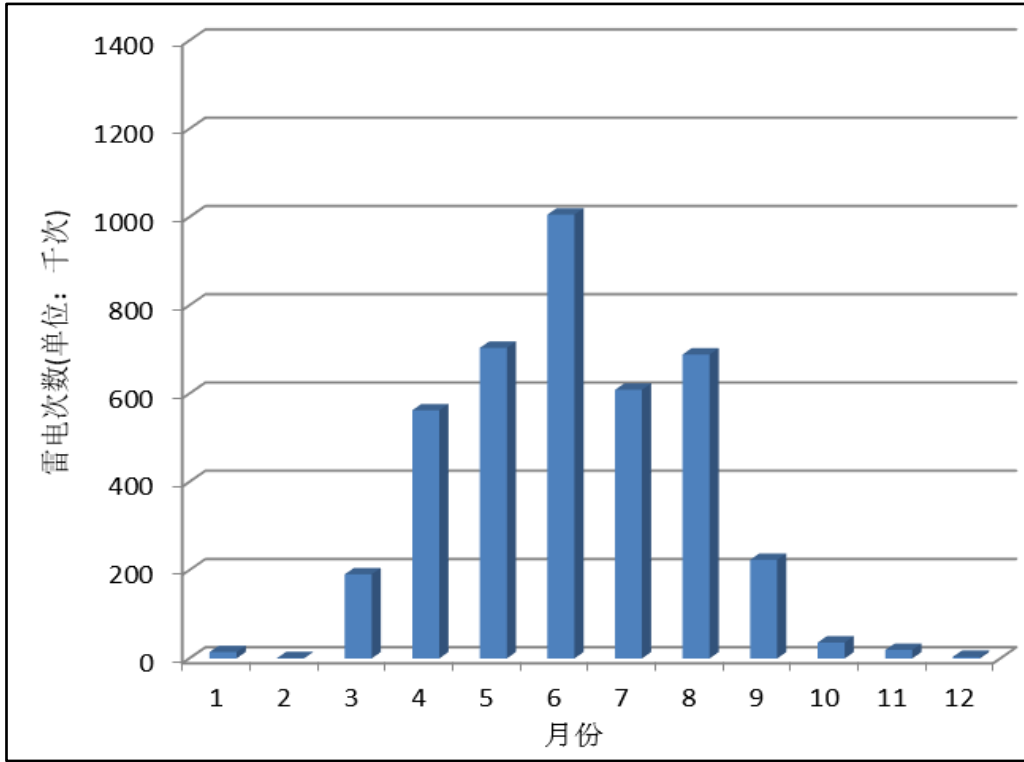
2016 年全省雷电活动月分布图
