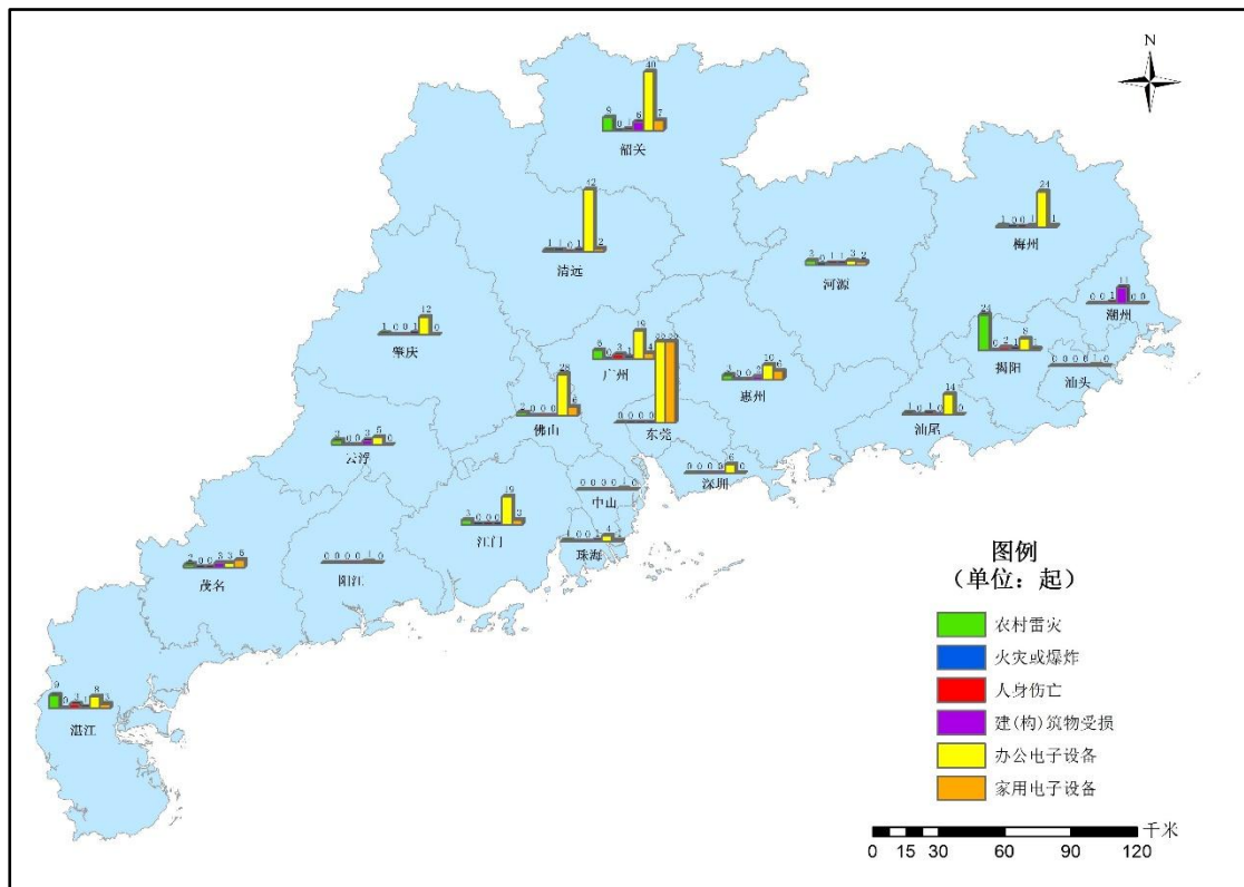
2016年各地市雷灾空间分布图
